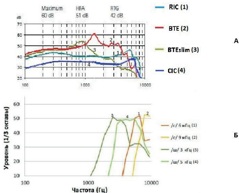
Рис. 6. А. Амплитудно-частотная характеристика аппаратов, применяемых в исследовании. Б. Спектральная форма звуков «с» и «ш», где пик — центральная часть фонемы
