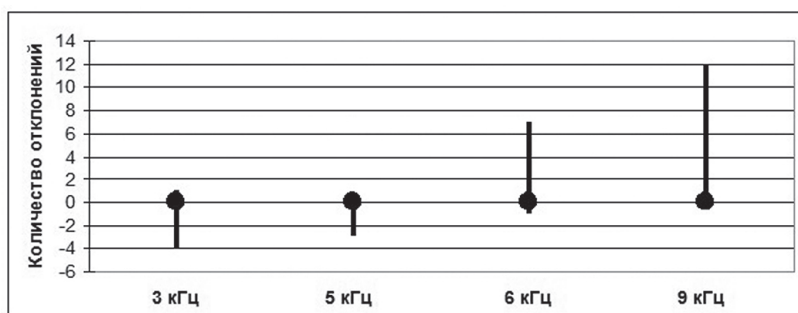
Рис. 3. Направленность отклонений в тесте обнаружения без слухового аппарата после 3-месячной адаптации
